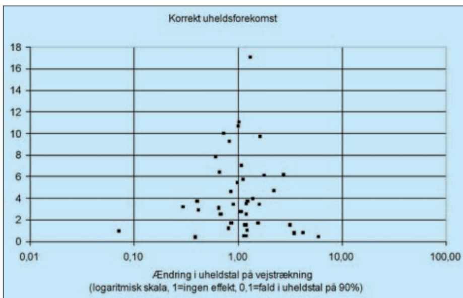
Figur 2. Funnelploj af uheldstal fra korrekt uheldsforekomst. Vægtet middeleffekt er 1,05, altså en stigning i uheld på 5%. Der er et 95% konfidensinterval på 0,91-1,22.
