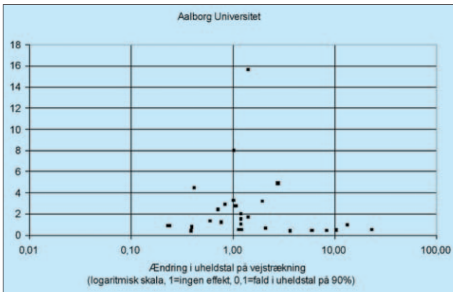
Figur 1. Funnelploj af uheldstal fra Aalborg Universitet. Vægtet middeleffekt er 1,23, altså en stigning i uheld på 23%. Der er et 95% konfidensinterval på 0,97-1,55.
