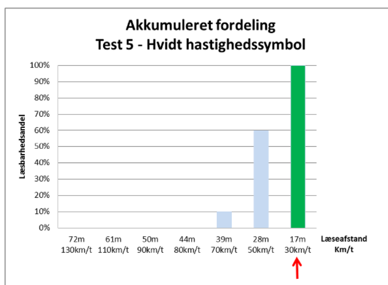
Figur 4.10: Kravet til læsbarhed af hvidt hastighedssymbol med H = 2,4 \text{ m} er opfyldt ved hastighedsniveauet på 30 km/t
