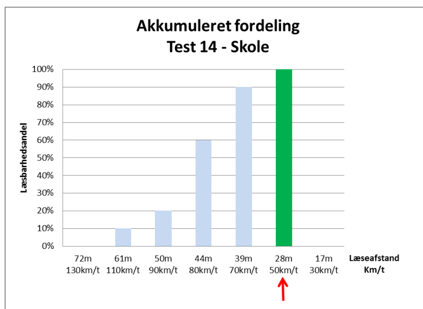
Figur 4.28: Kravet om tilstrækkelig læsbarhed af teksten "Skole" med H = 1,6 m er opfyldt ved hastighedsniveau på 50 km/t.
