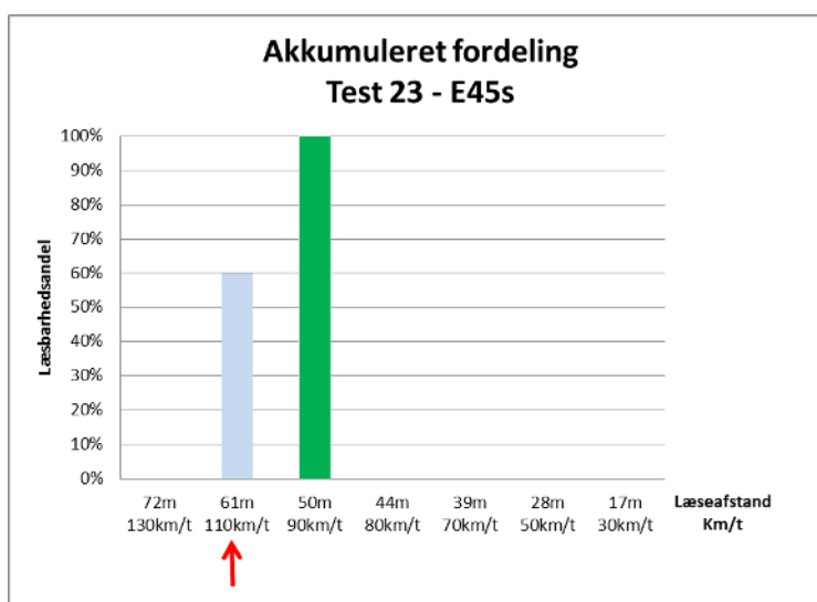
Figur 4.46: Kravet om tilstrækkelig læsbarhed af den samlede information er ikke opfyldt ved hastighedsniveau på 110 km/t, fordi lille "s" ikke er tilstrækkelig læsbart i afstand på 61 m.
